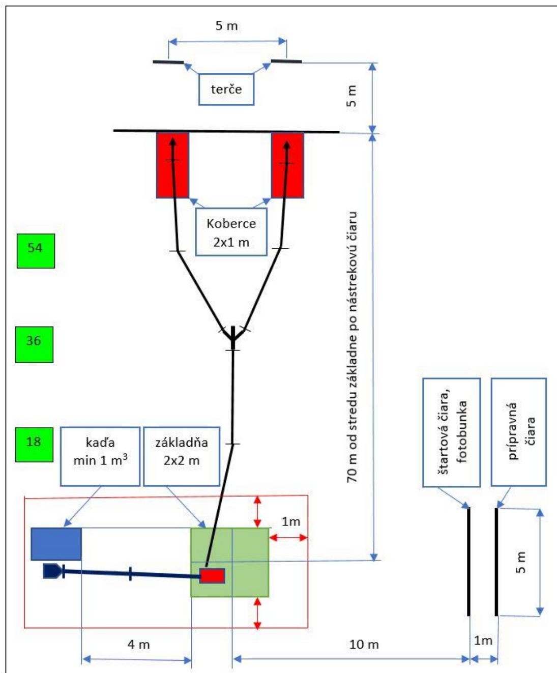
Obr. 3.1 - Schéma a plánik trate
